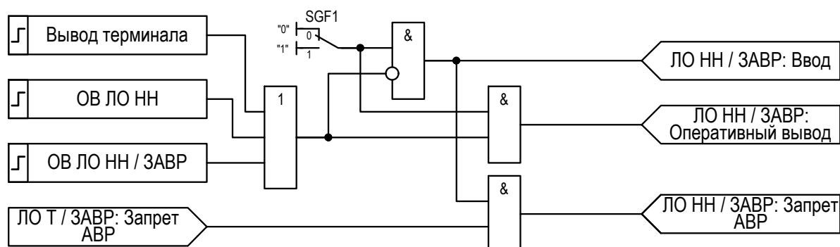
Рисунок 2.27 – Функциональная схема «Запрет АБР»
