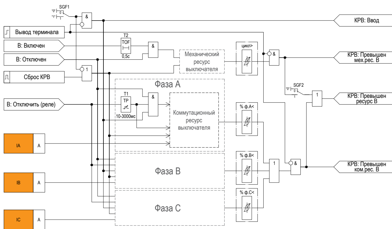
Рисунок 2.29 – Функциональная схема «КРВ»
