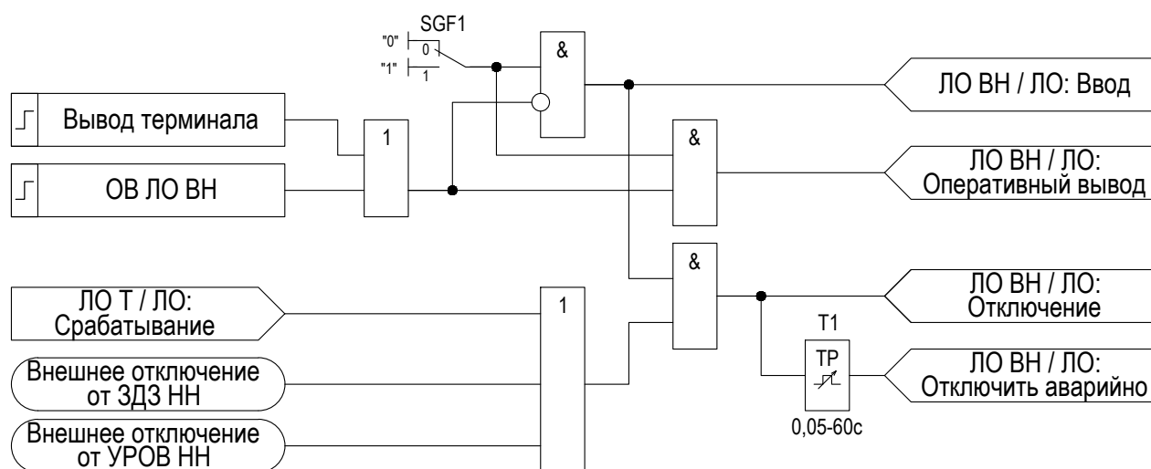
Рисунок 2.24 – Функциональная схема «ЛО»
